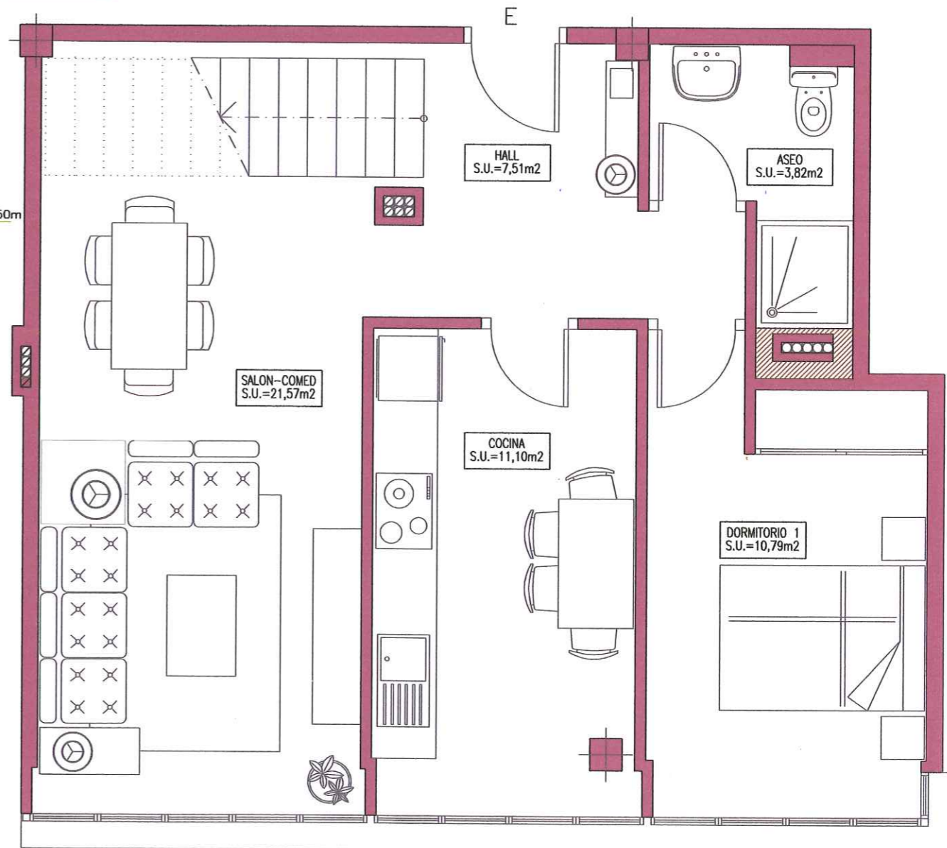
Planta Tercera
